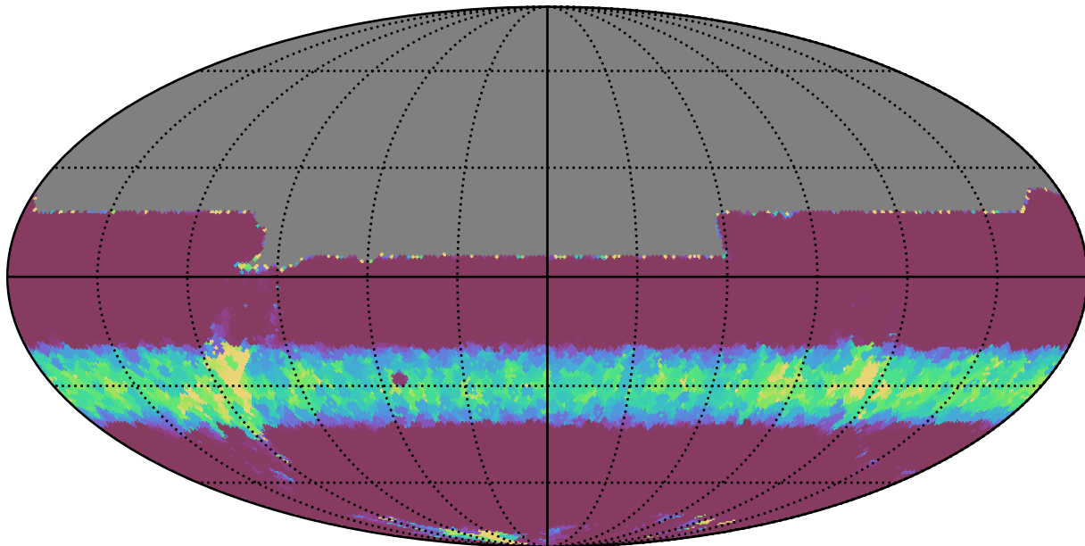
weather_cloudso20v3.4_10yrs All sky y band: Min normairmass
