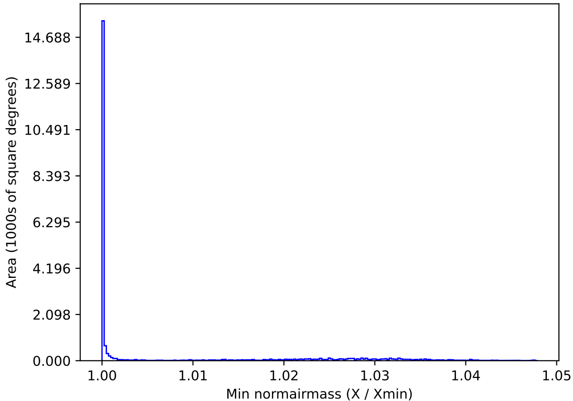
weather_cloudso20v3.4_10yrs All sky y band: Min normairmass
