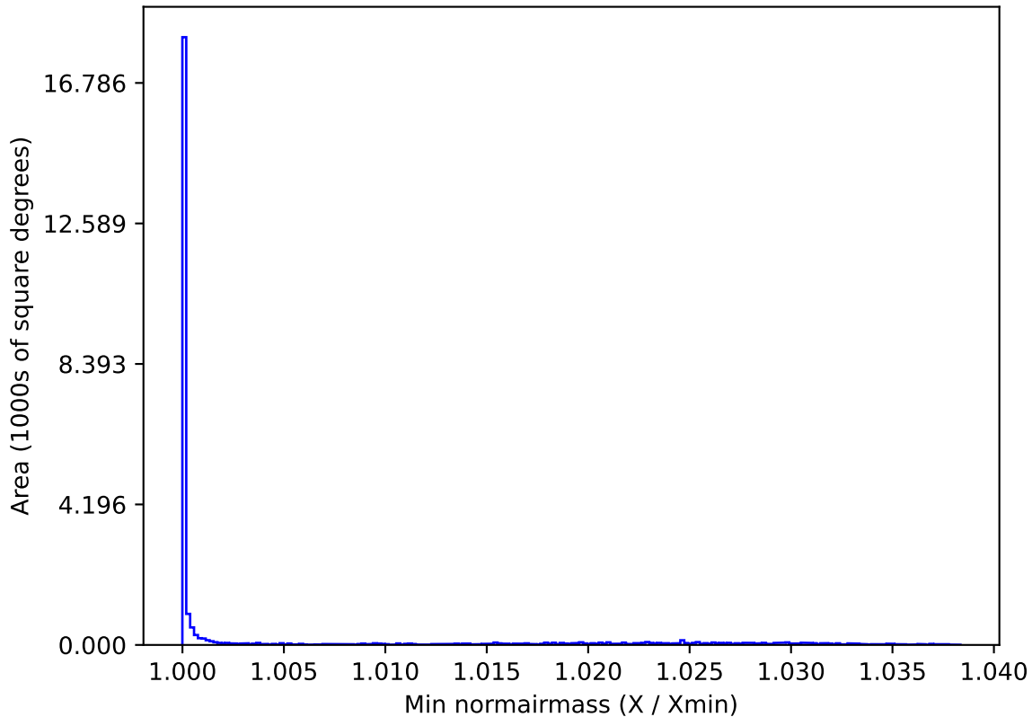
weather_cloudso20v3.4_10yrs All sky r band: Min normairmass
