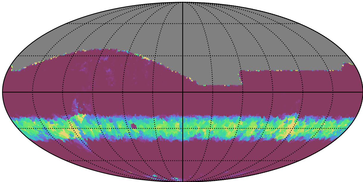
weather_cloudso20v3.4_10yrs All sky i band: Min normairmass
