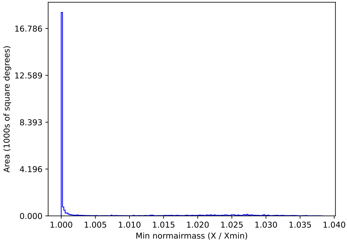
weather_cloudso20v3.4_10yrs All sky i band: Min normairmass
