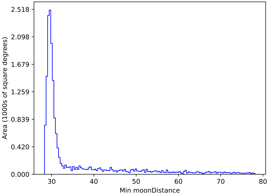
weather_cloudso20v3.4_10yrs WFD z band: Min moonDistance
