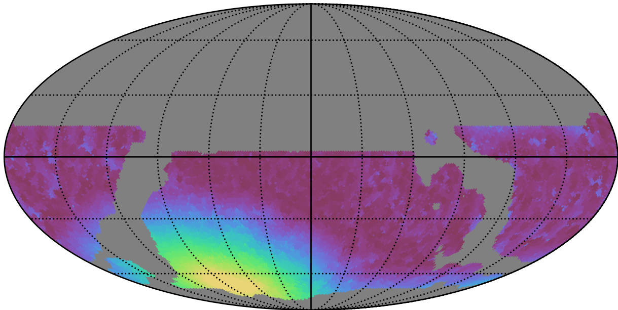
weather_cloudso20v3.4_10yrs WFD r band: Min moonDistance
