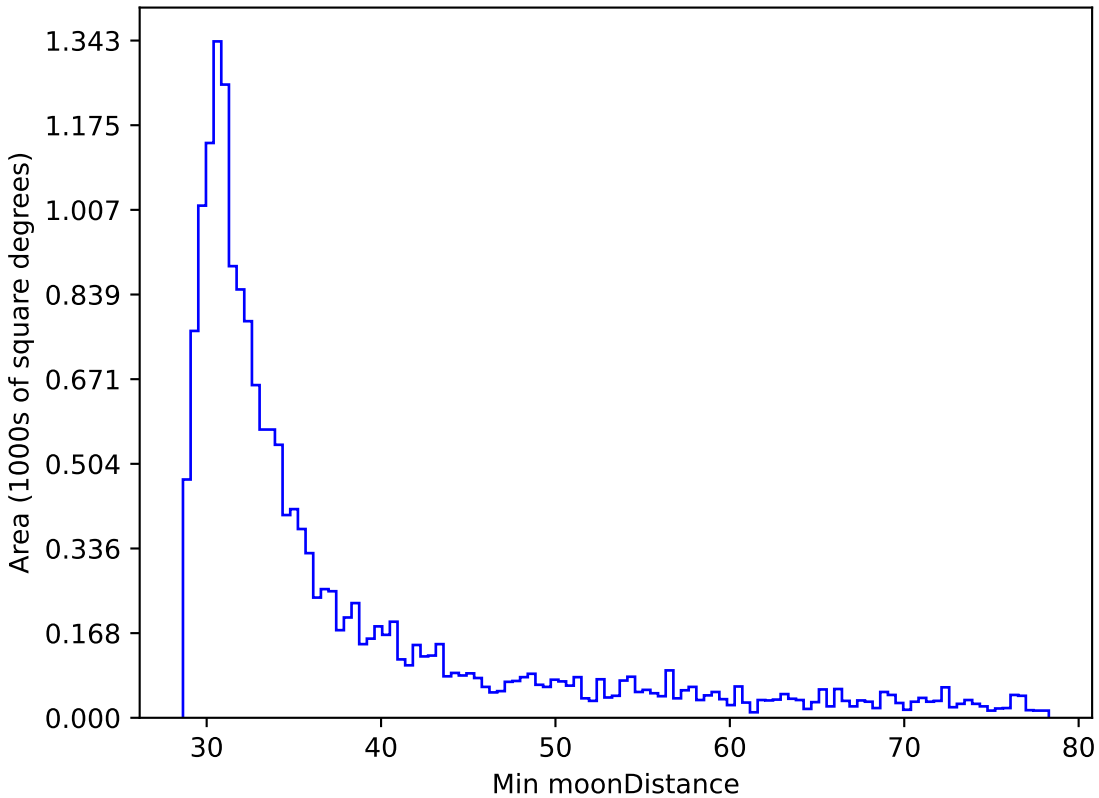
weather_cloudso20v3.4_10yrs WFD r band: Min moonDistance
