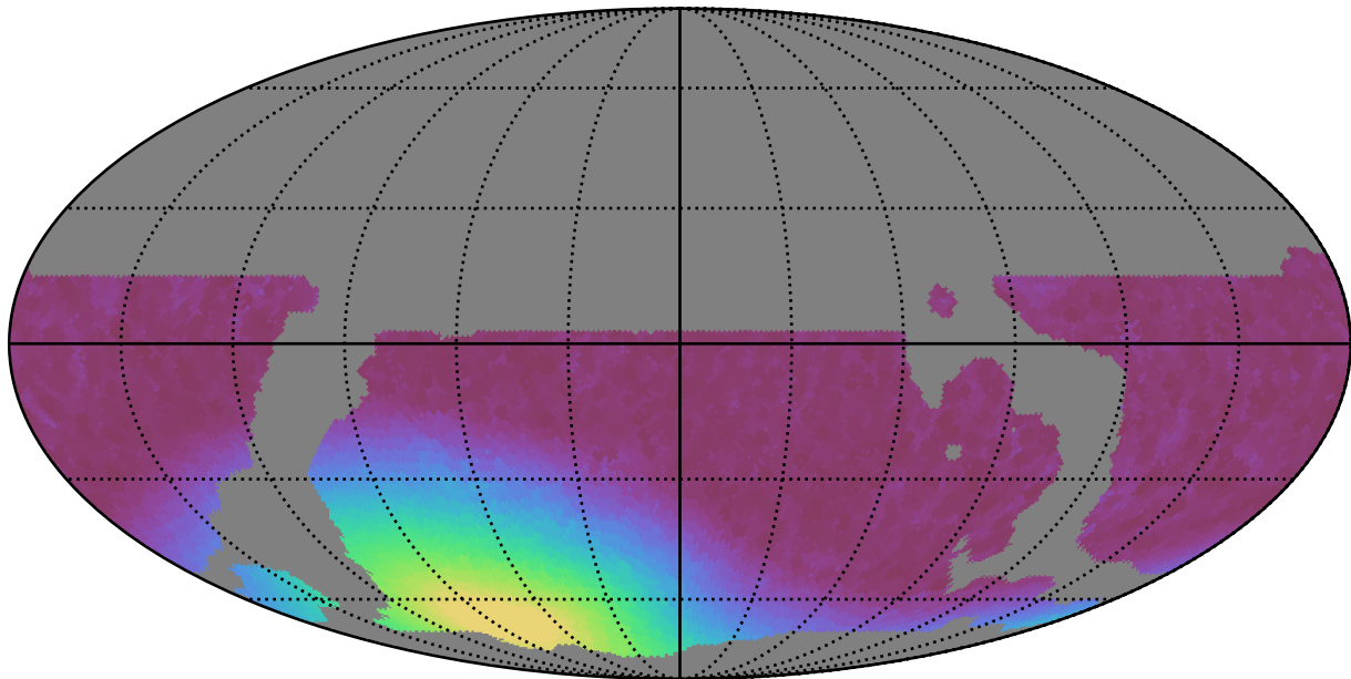
weather_cloudso20v3.4_10yrs WFD i band: Min moonDistance
