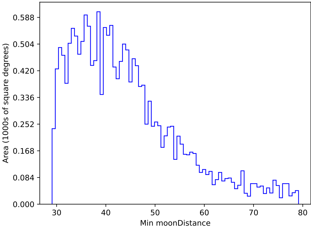
weather_cloudso20v3.4_10yrs WFD g band: Min moonDistance
