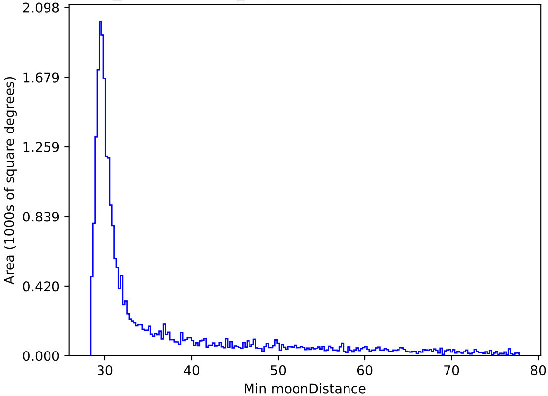
weather_cloudso20v3.4_10yrs All sky z band: Min moonDistance
