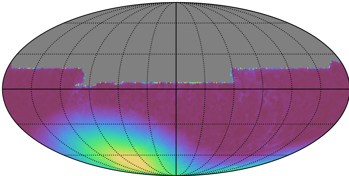
weather_cloudso20v3.4_10yrs All sky y band: Min moonDistance
