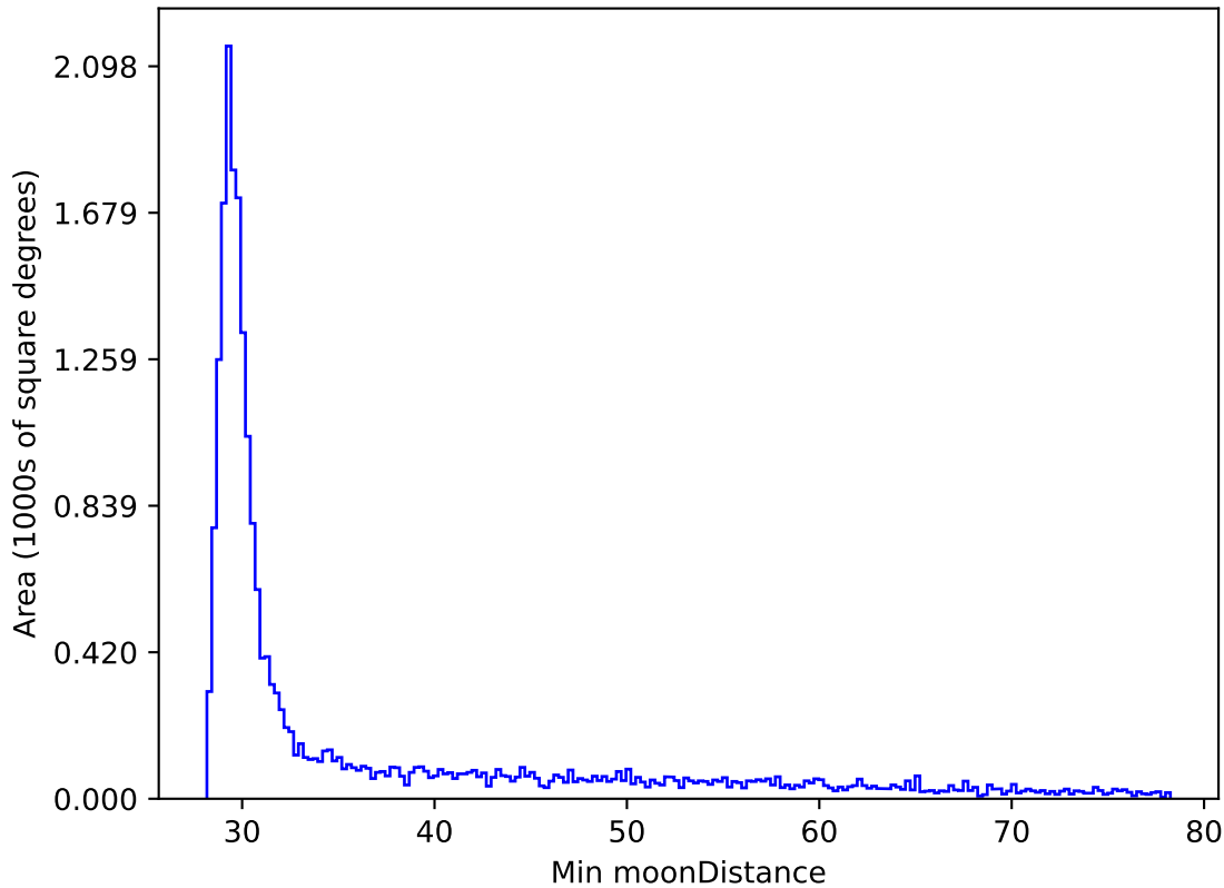
weather_cloudso20v3.4_10yrs All sky y band: Min moonDistance
