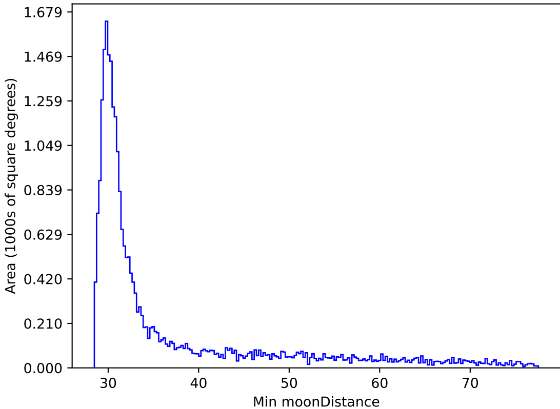
weather_cloudso20v3.4_10yrs All sky i band: Min moonDistance
