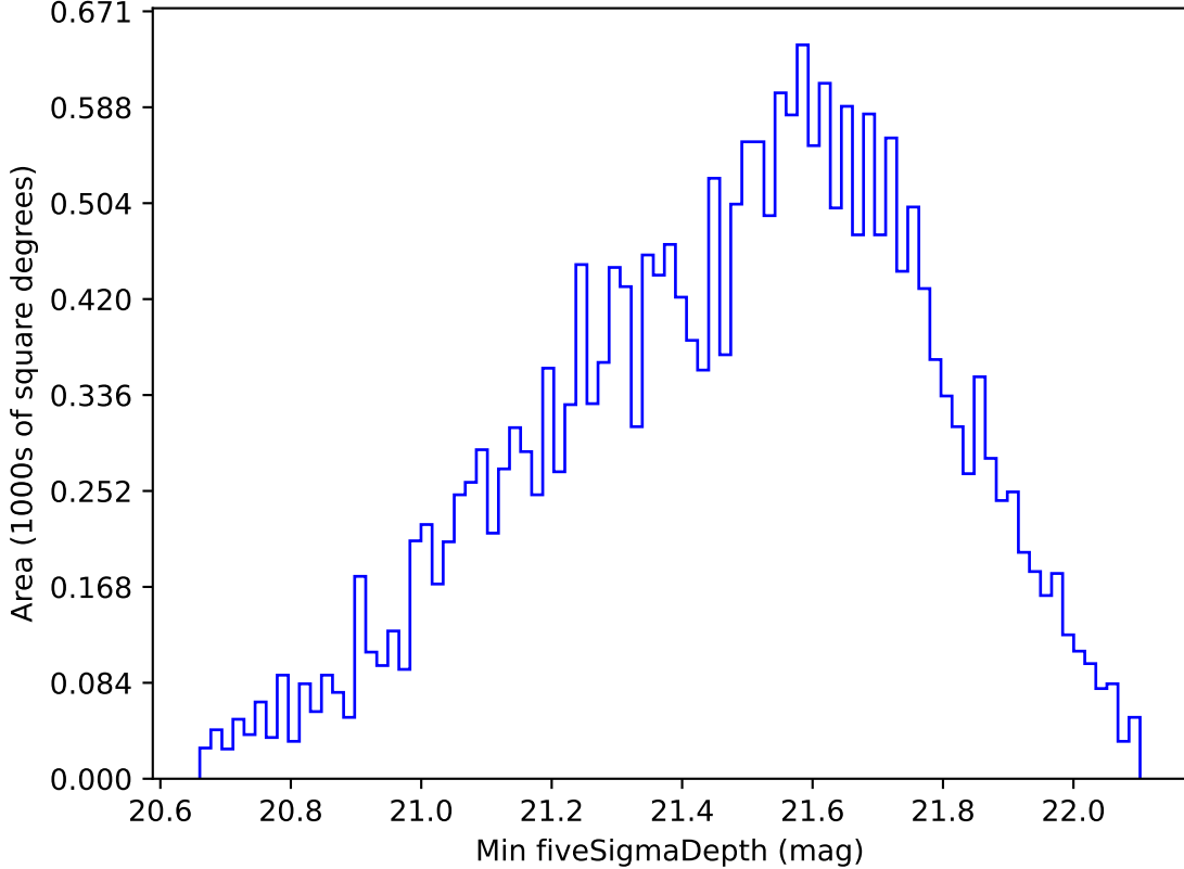
weather_cloudso20v3.4_10yrs Yr 1 y band: Min fiveSigmaDepth
