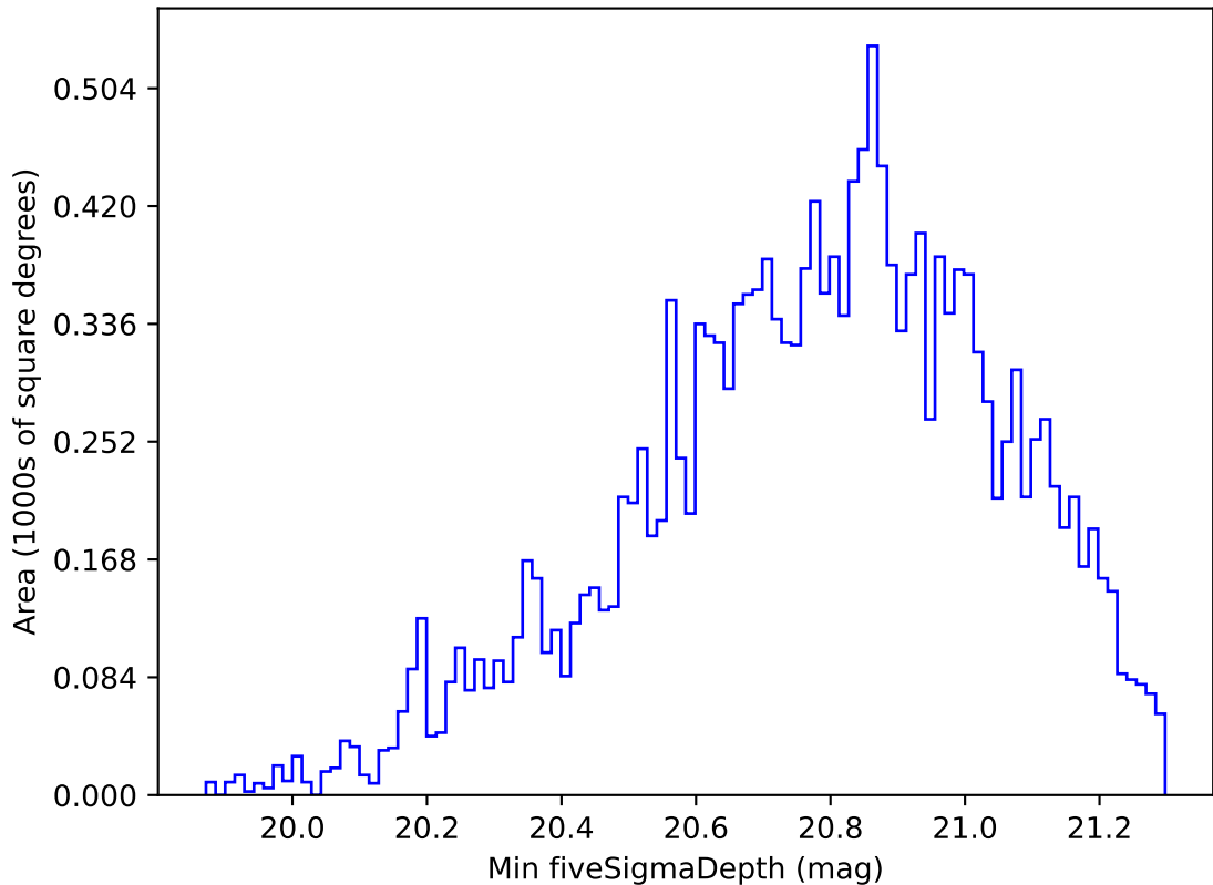
weather_cloudso20v3.4_10yrs WFD y band: Min fiveSigmaDepth
