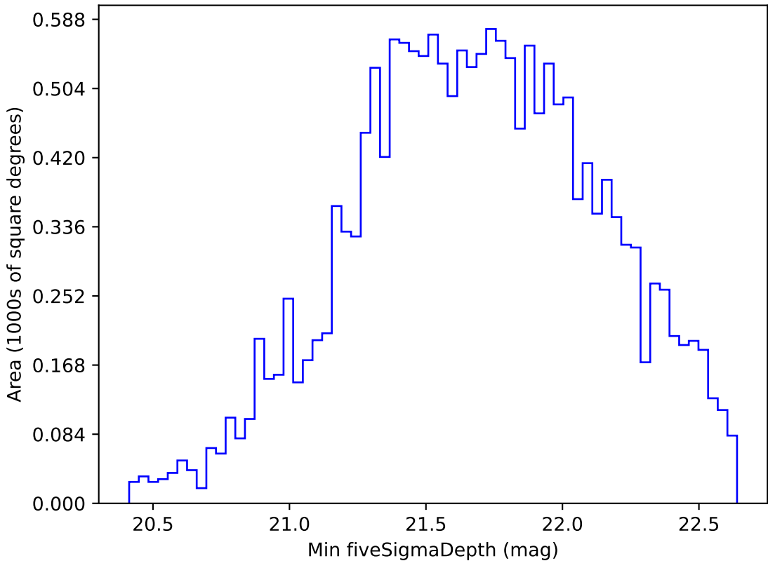
weather_cloudso20v3.4_10yrs WFD i band: Min fiveSigmaDepth
