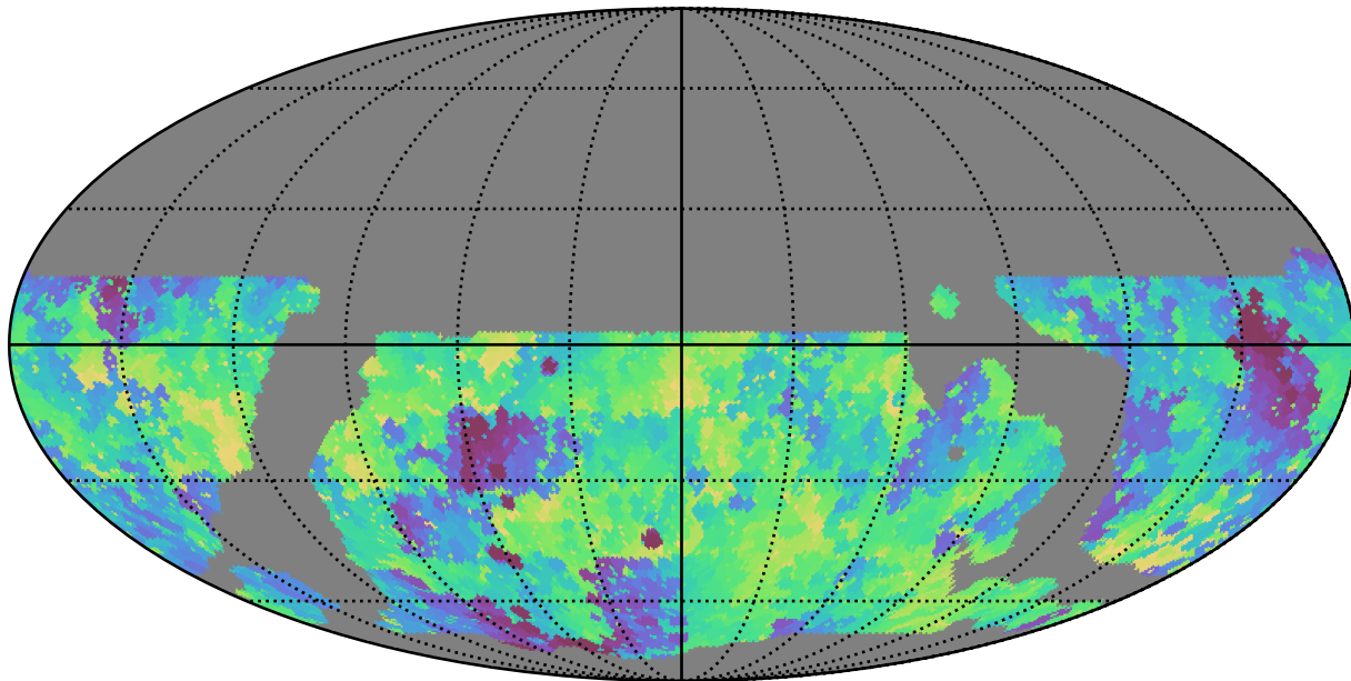
weather_cloudso20v3.4_10yrs WFD g band: Min fiveSigmaDepth
