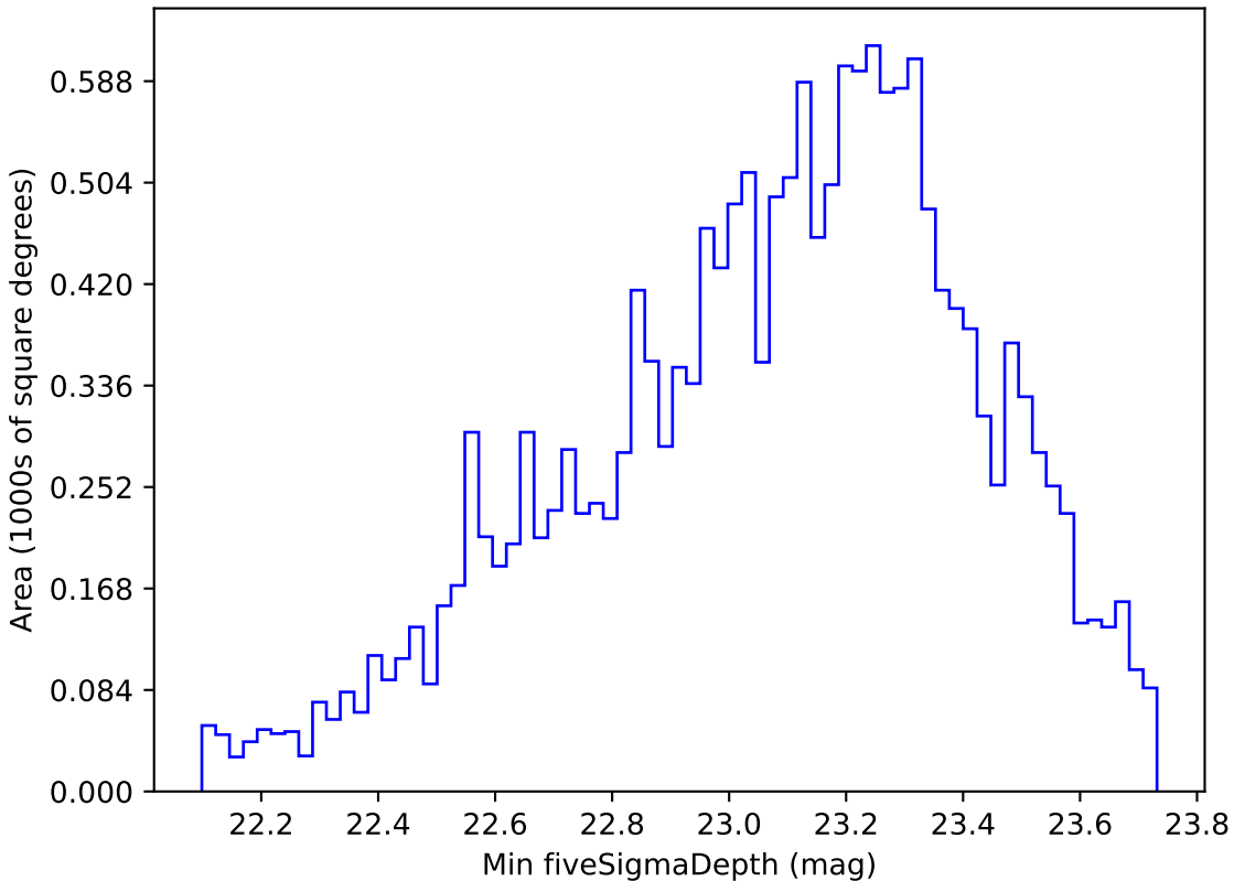
weather_cloudso20v3.4_10yrs WFD g band: Min fiveSigmaDepth
