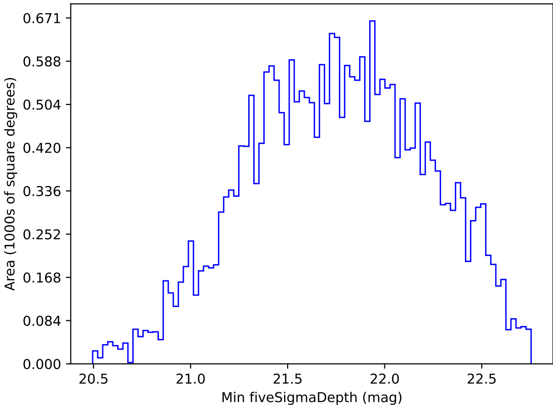
weather_cloudso20v3.4_10yrs All sky i band: Min fiveSigmaDepth
