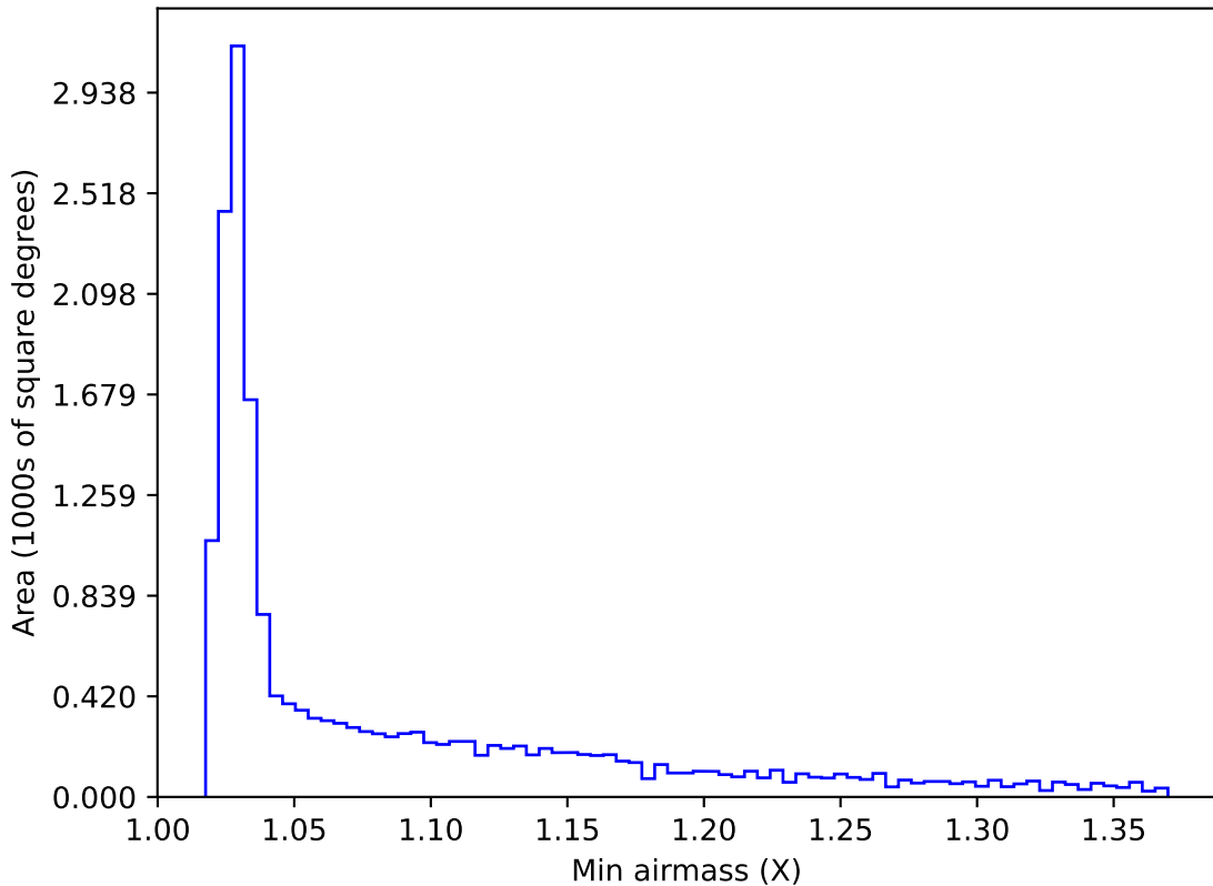
weather_cloudso20v3.4_10yrs WFD i band: Min airmass
