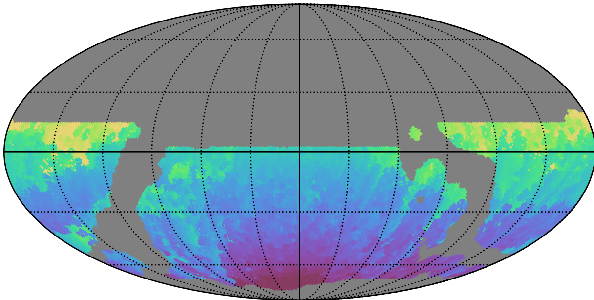
weather_cloudso20v3.4_10yrs WFD z band: Min HA
