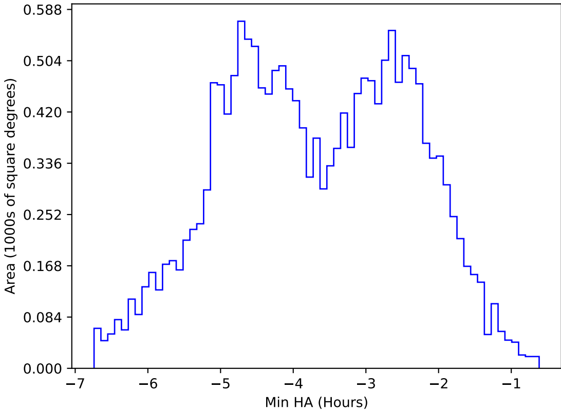
weather_cloudso20v3.4_10yrs WFD y band: Min HA
