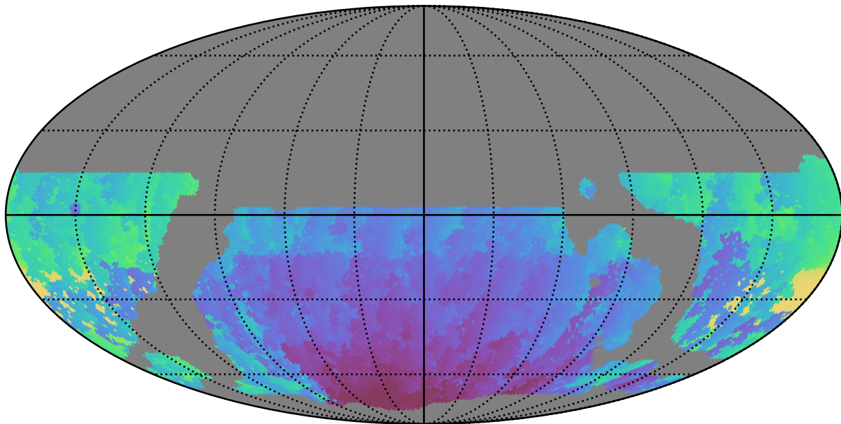
weather_cloudso20v3.4_10yrs WFD u band: Min HA
