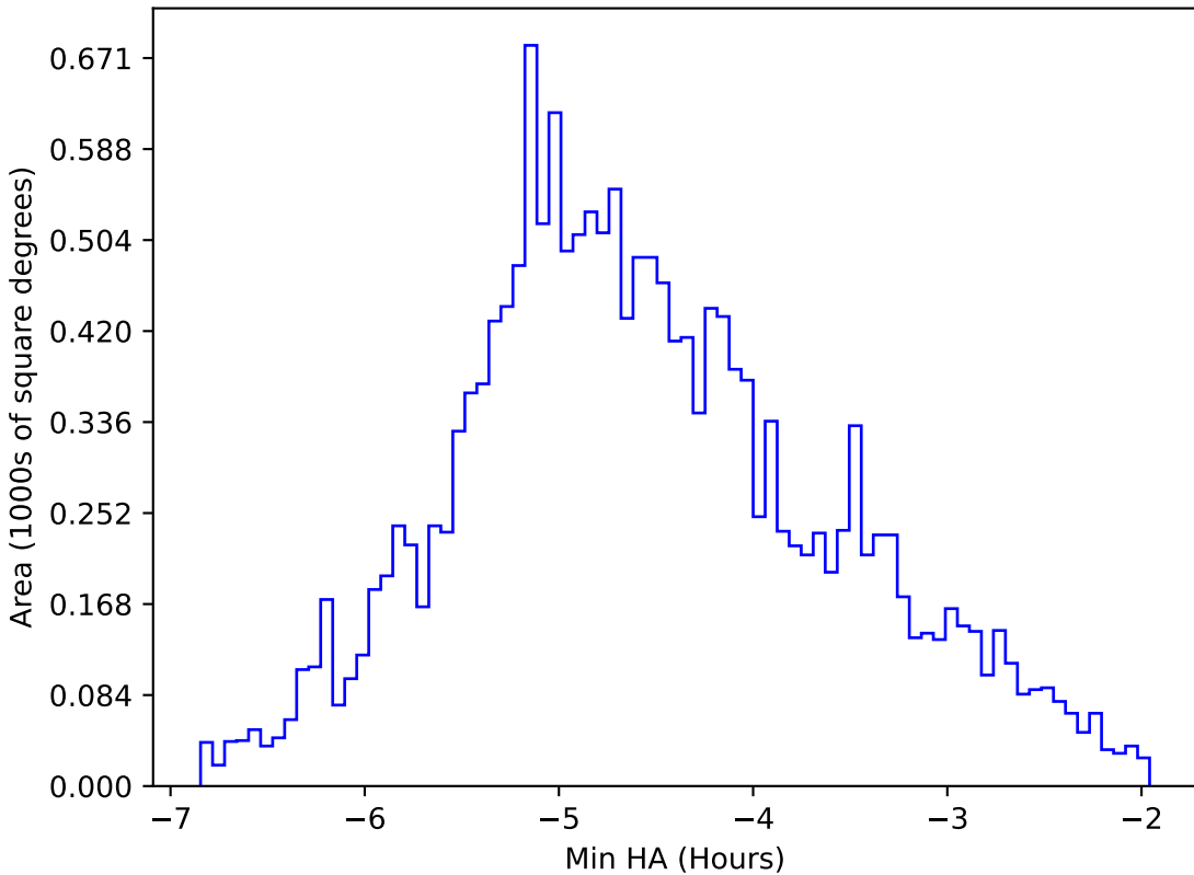
weather_cloudso20v3.4_10yrs WFD r band: Min HA
