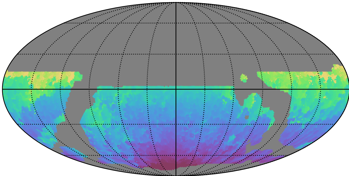
weather_cloudso20v3.4_10yrs WFD i band: Min HA
