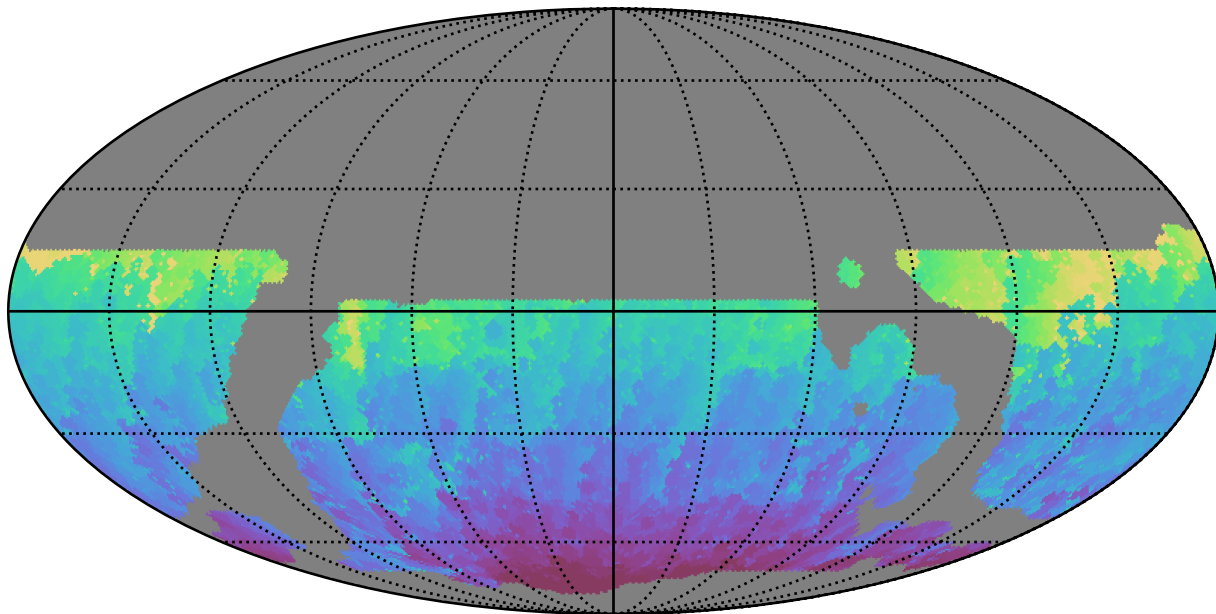
weather_cloudso20v3.4_10yrs WFD g band: Min HA
