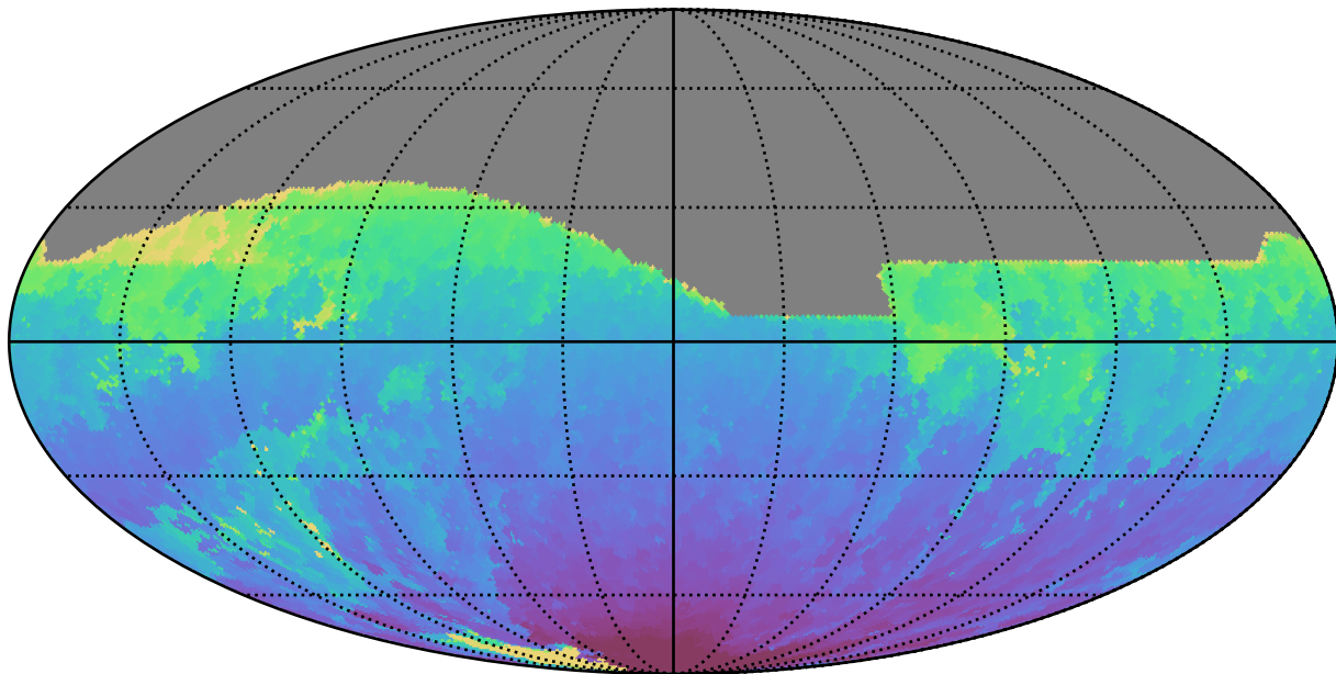
weather_cloudso20v3.4_10yrs All sky z band: Min HA
