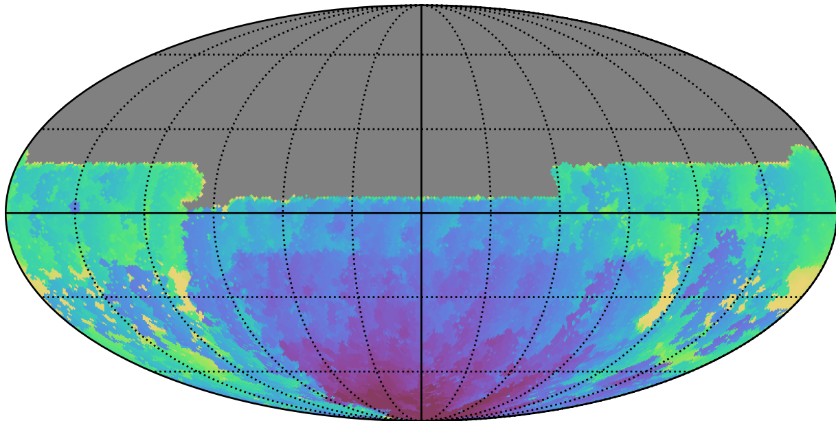
weather_cloudso20v3.4_10yrs All sky u band: Min HA
