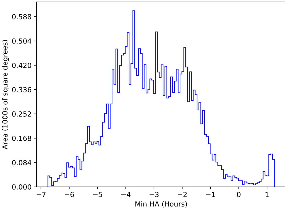
weather_cloudso20v3.4_10yrs All sky u band: Min HA
