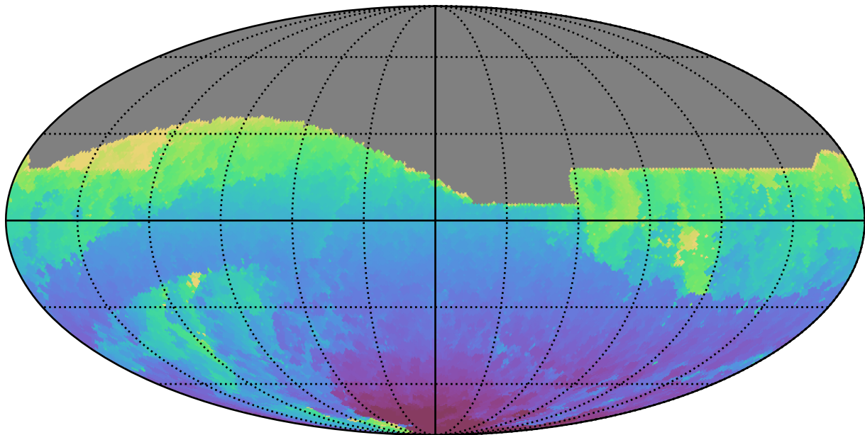
weather_cloudso20v3.4_10yrs All sky r band: Min HA
