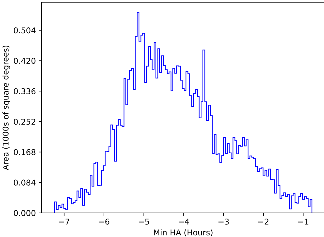
weather_cloudso20v3.4_10yrs All sky r band: Min HA
