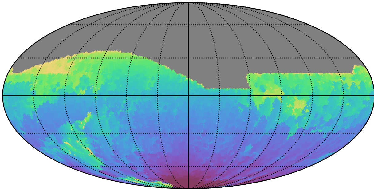
weather_cloudso20v3.4_10yrs All sky i band: Min HA
