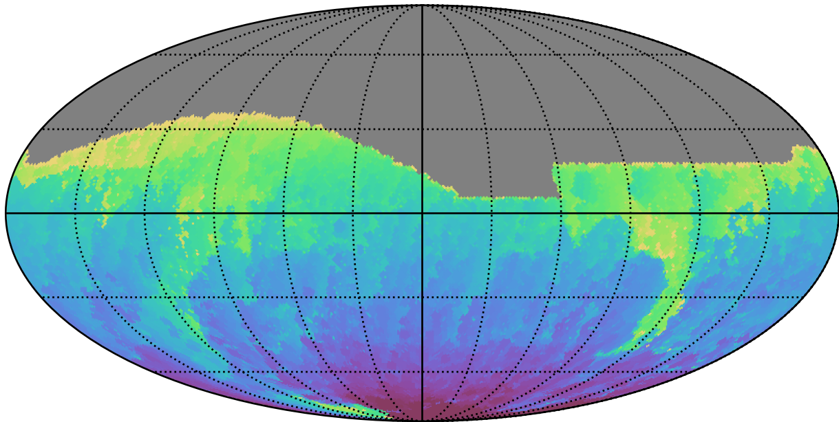
weather_cloudso20v3.4_10yrs All sky g band: Min HA
