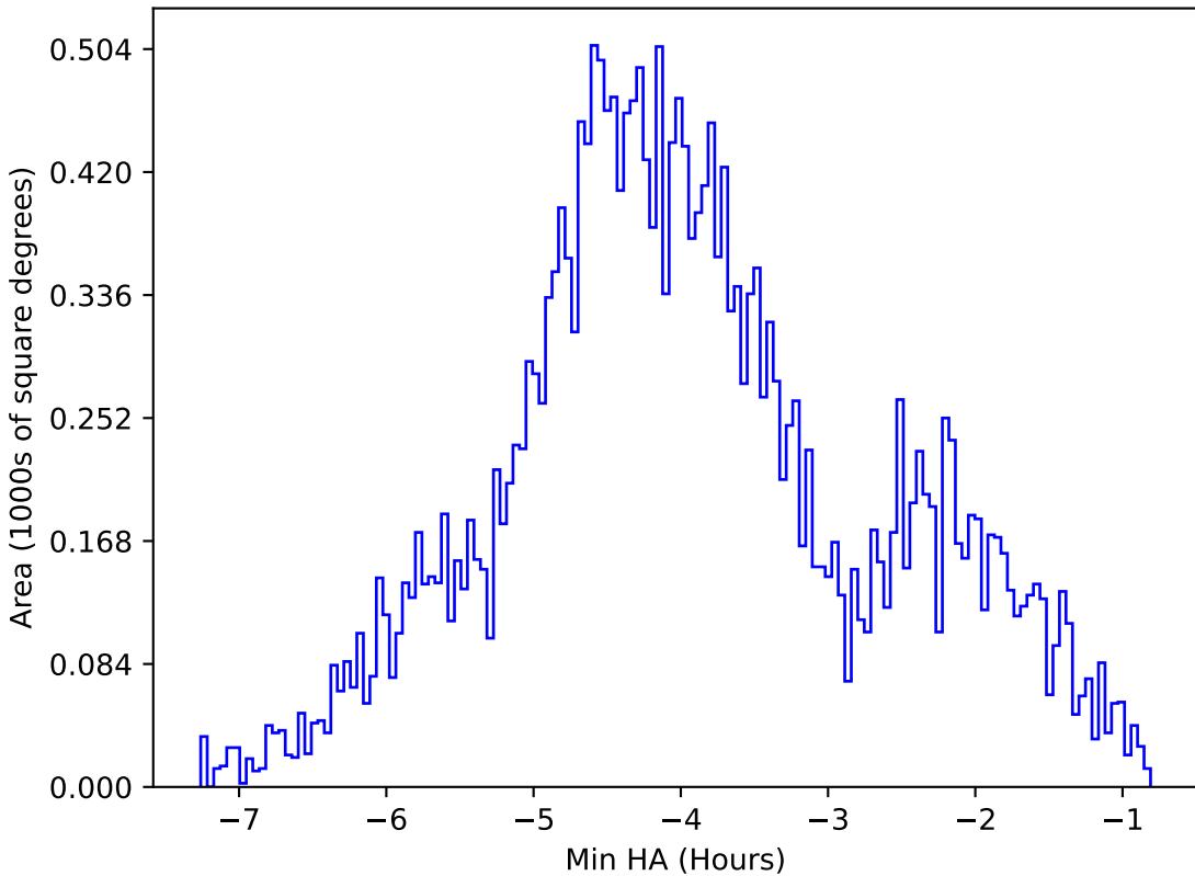
weather_cloudso20v3.4_10yrs All sky g band: Min HA
