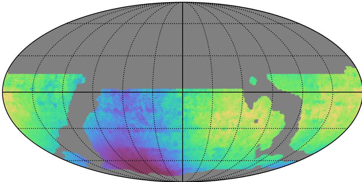
weather_cloudso20v3.4_10yrs WFD z band: Median solarElong
