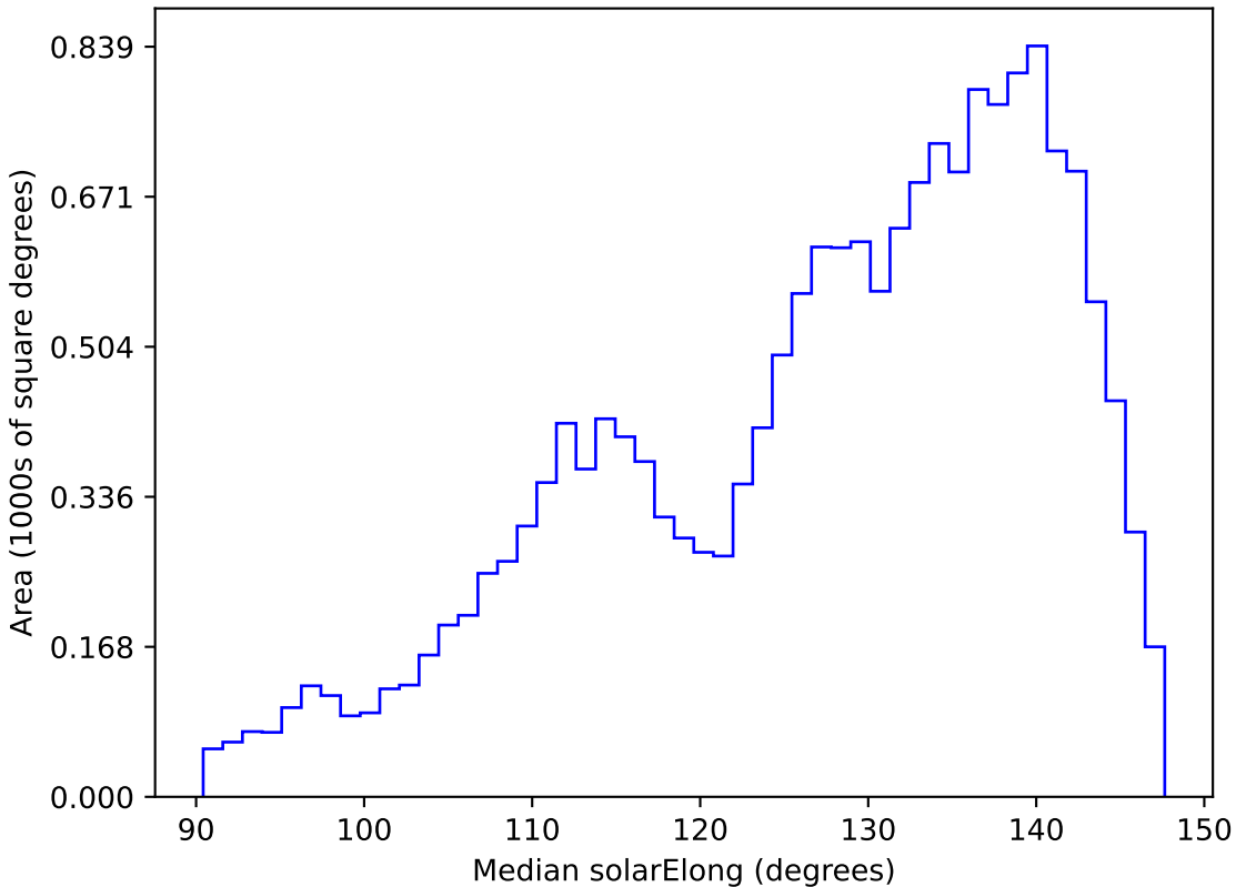
weather_cloudso20v3.4_10yrs WFD z band: Median solarElong
