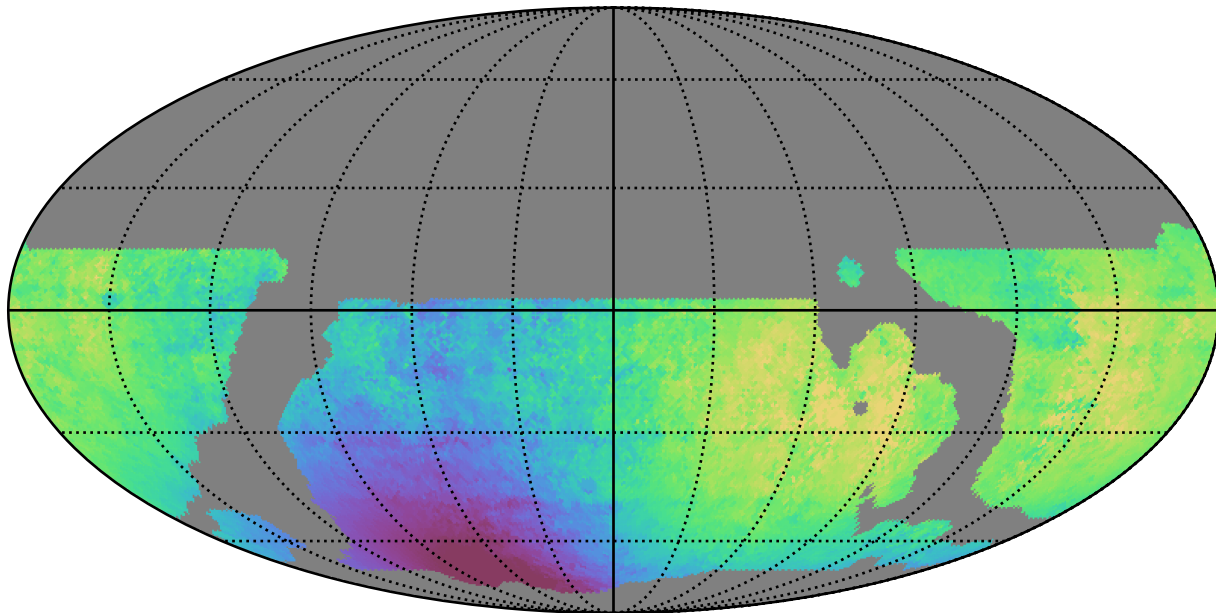
weather_cloudso20v3.4_10yrs WFD y band: Median solarElong
