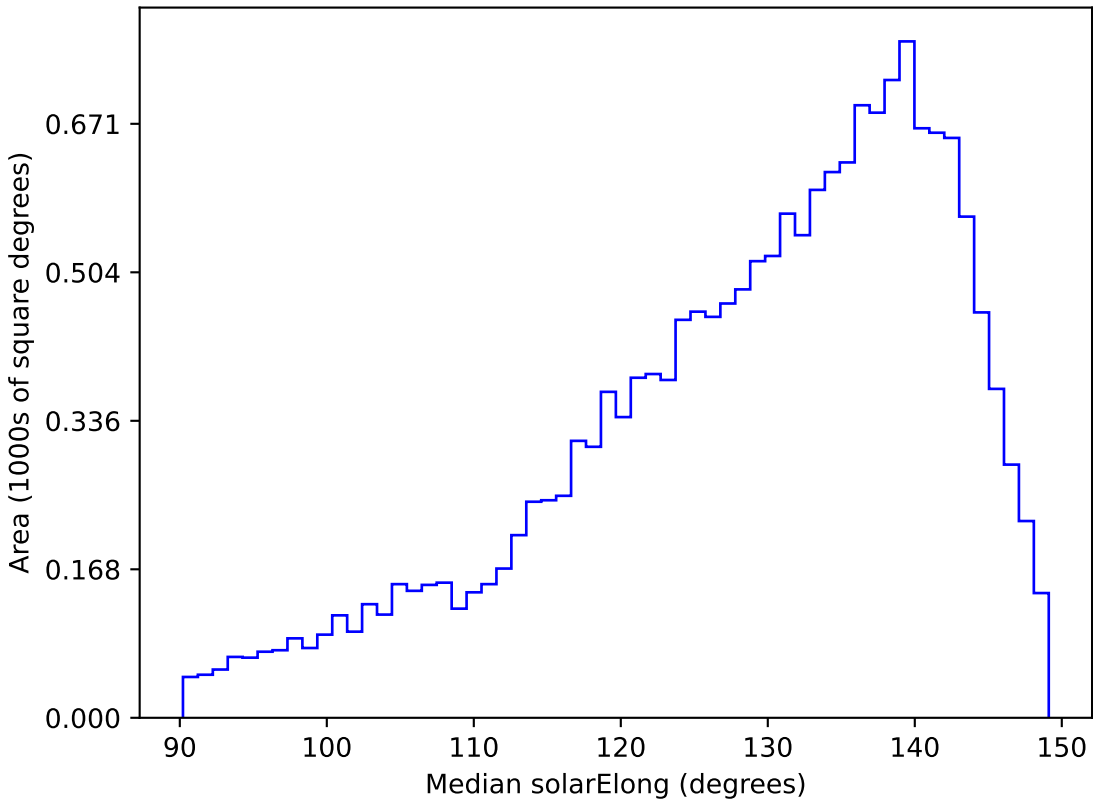
weather_cloudso20v3.4_10yrs WFD y band: Median solarElong
