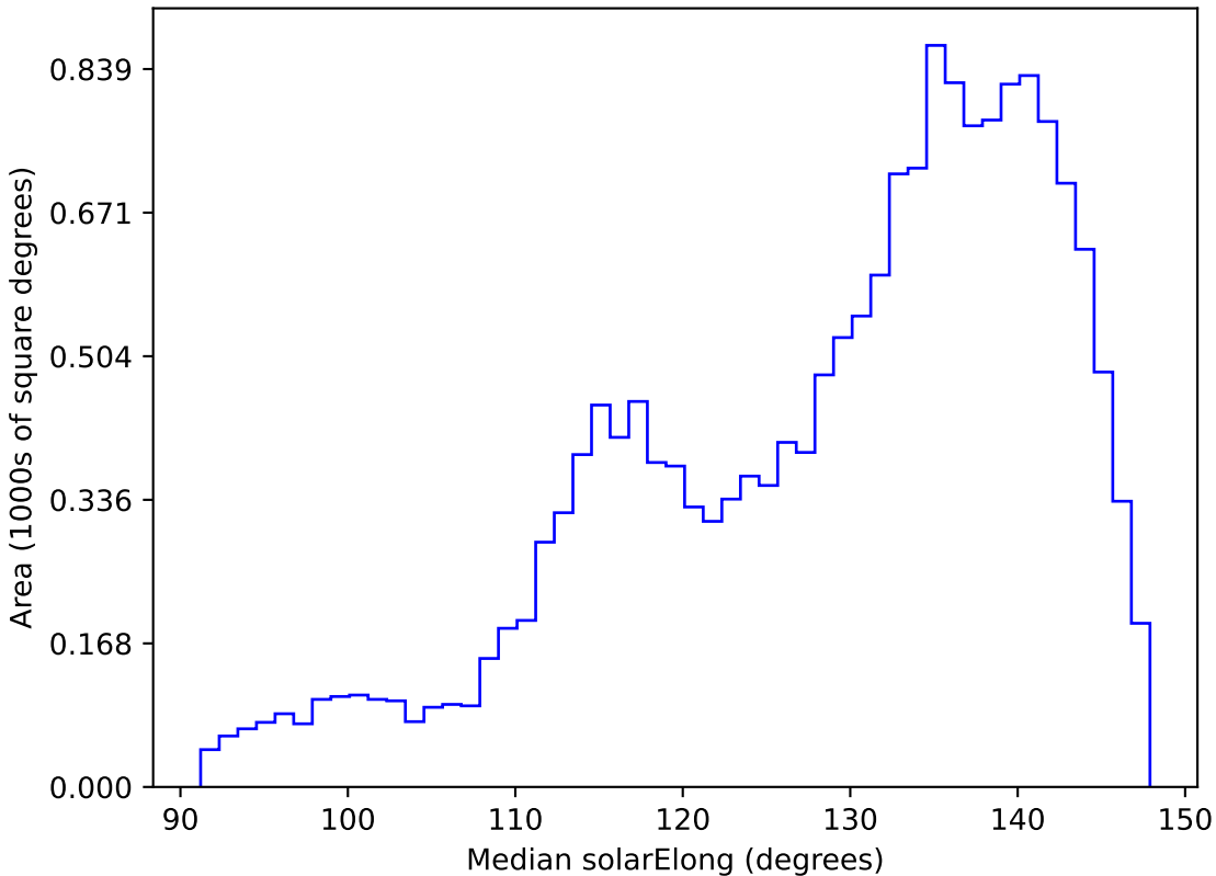
weather_cloudso20v3.4_10yrs WFD i band: Median solarElong
