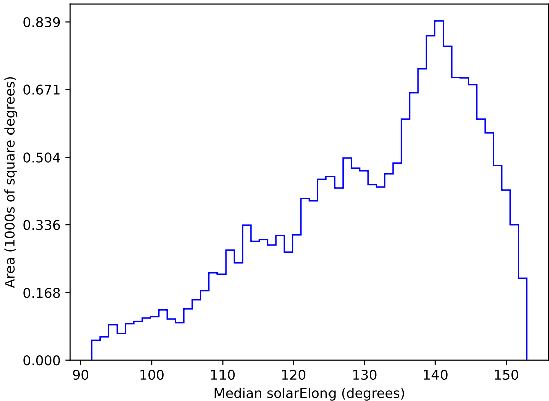
weather_cloudso20v3.4_10yrs WFD g band: Median solarElong
