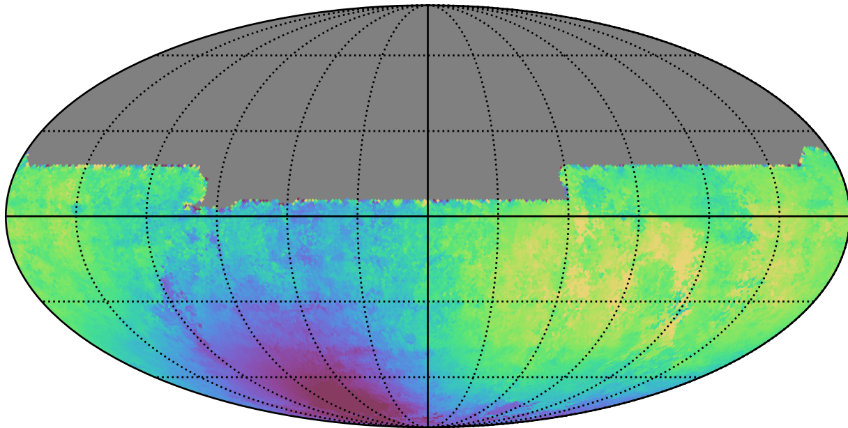
weather_cloudso20v3.4_10yrs All sky y band: Median solarElong
