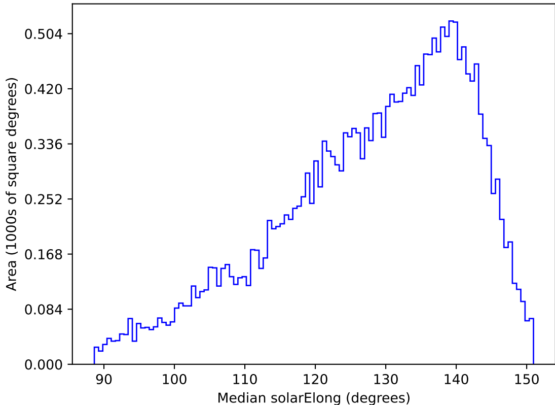
weather_cloudso20v3.4_10yrs All sky y band: Median solarElong
