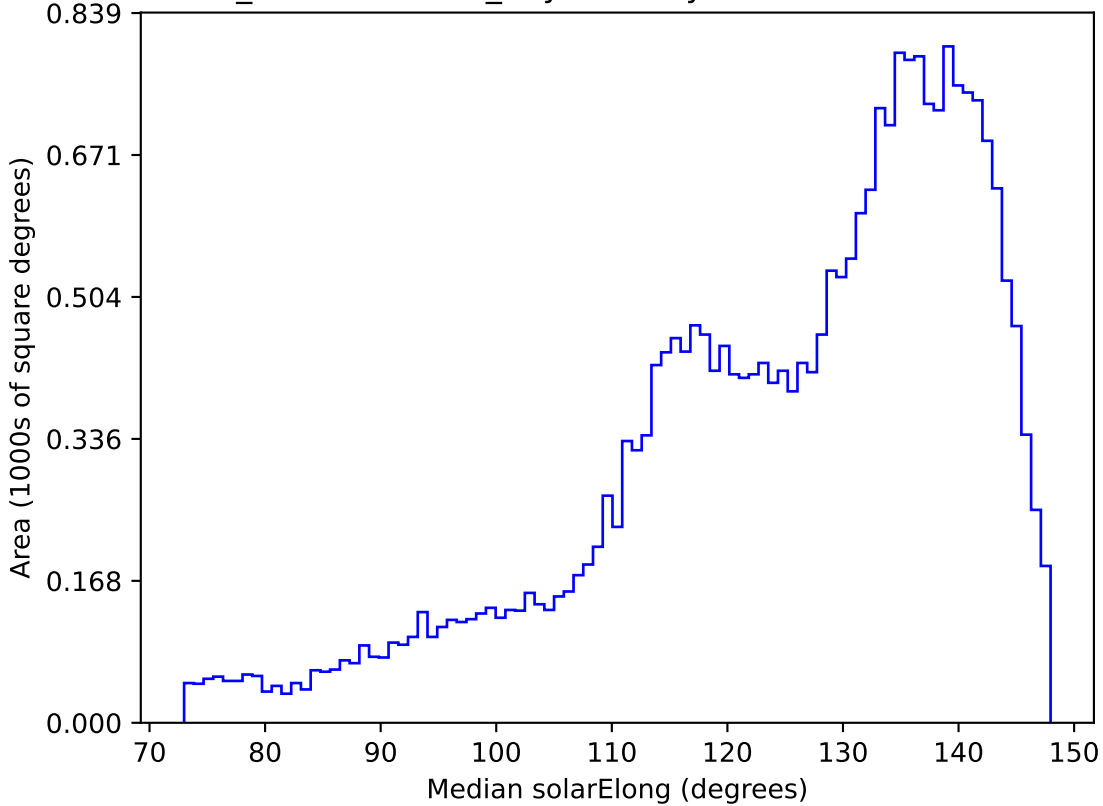
weather_cloudso20v3.4_10yrs All sky i band: Median solarElong
