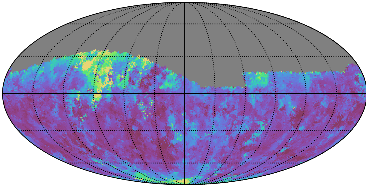
weather_cloudso20v3.4_10yrs Yr 1 z band: Median seeingGeom
