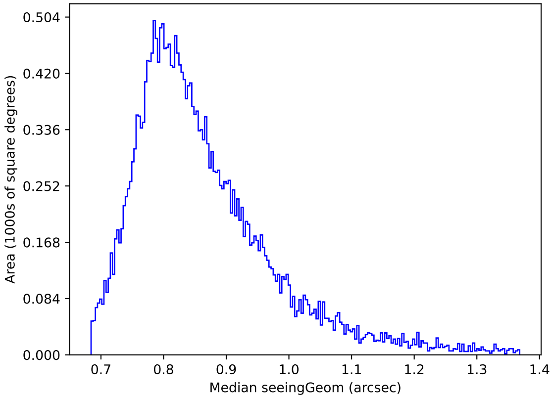
weather_cloudso20v3.4_10yrs Yr 1 z band: Median seeingGeom
