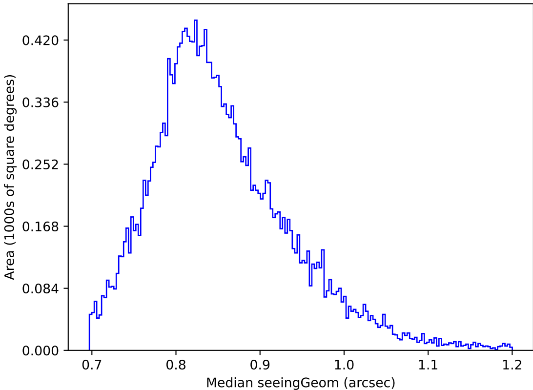
weather_cloudso20v3.4_10yrs Yr 1 y band: Median seeingGeom
