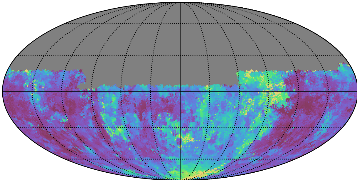
weather_cloudso20v3.4_10yrs Yr 1 u band: Median seeingGeom
