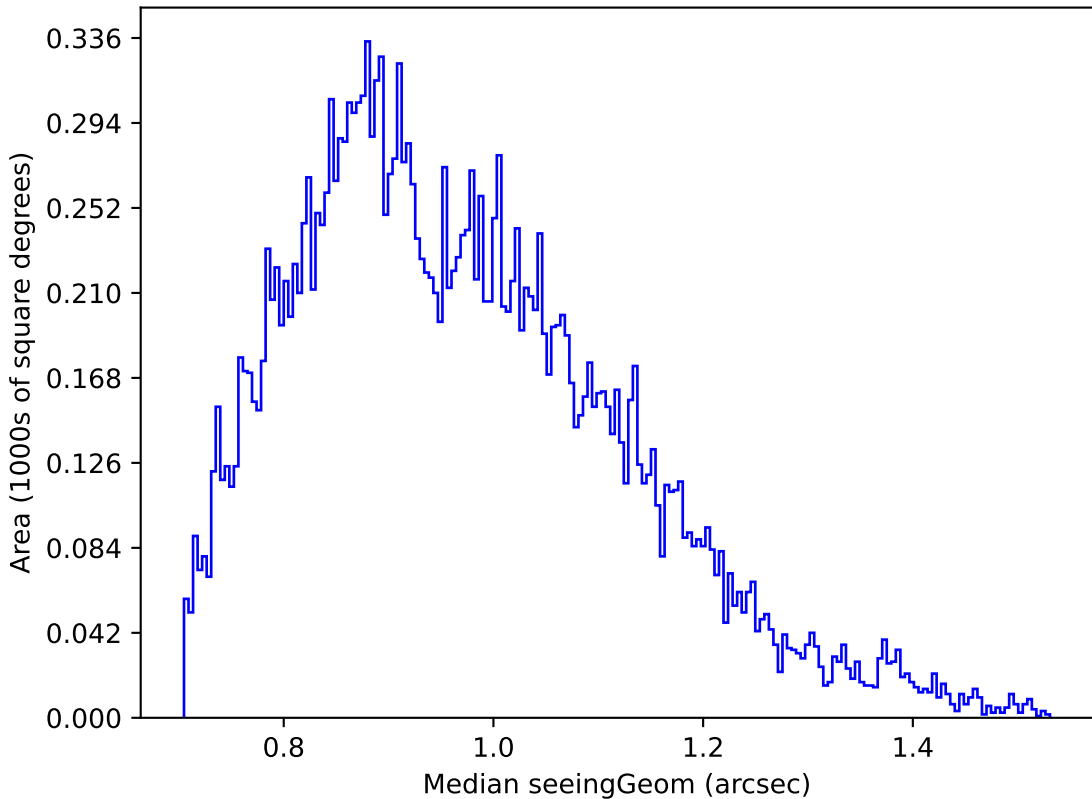
weather_cloudso20v3.4_10yrs Yr 1 u band: Median seeingGeom
