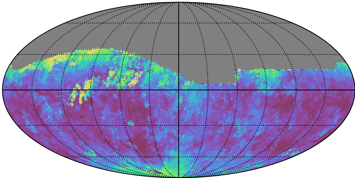
weather_cloudso20v3.4_10yrs Yr 1 r band: Median seeingGeom
